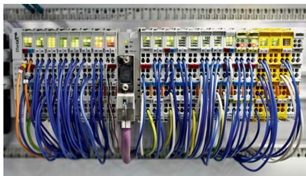
生产线上的所有安全设备，包括传送路径上的全部急停按钮，都可以通过集成到倍福 I/O 系统中的 TwinSAFE 端子模块来进行操作
