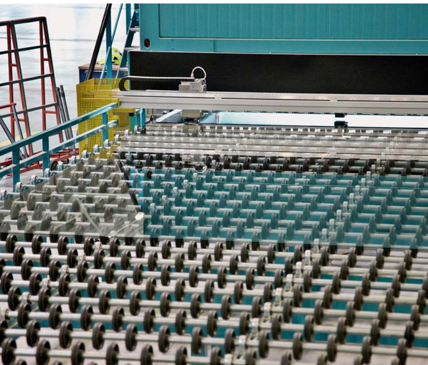
涂层处理之后的质量控制。在电阻测量之前，光学传感器会测量玻璃板的反射光与透射光
