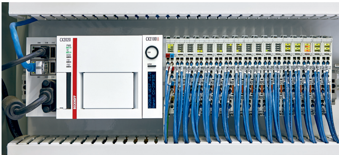
泵站通过直接插接 EtherCAT I/O 的 CX2020 嵌入式控制器控制
